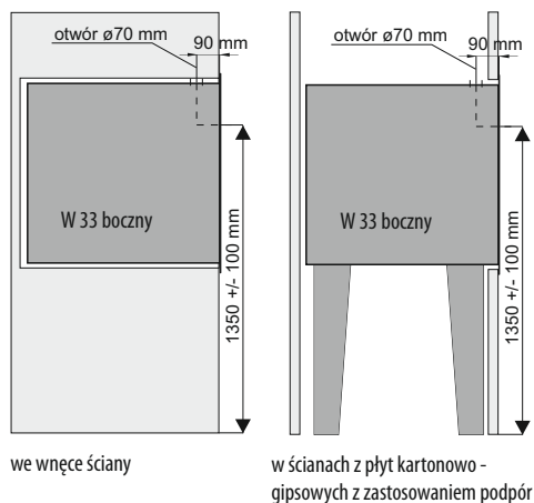
Rys. 2 Hydrant włączkowy
