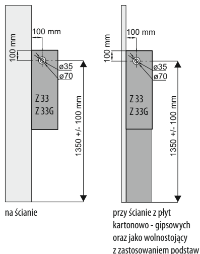
Rys. 1 Hydrant zawieszany
