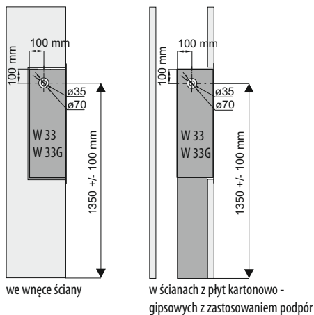
Rys. 2 Hydrant włączkowy
