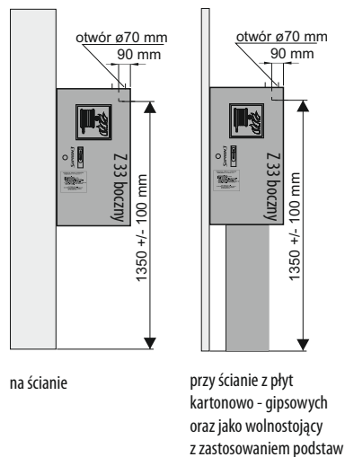
Rys. 1 Hydrant zawieszany
