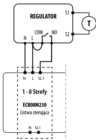
c) Schemat podłączenia do listwy sterującej
