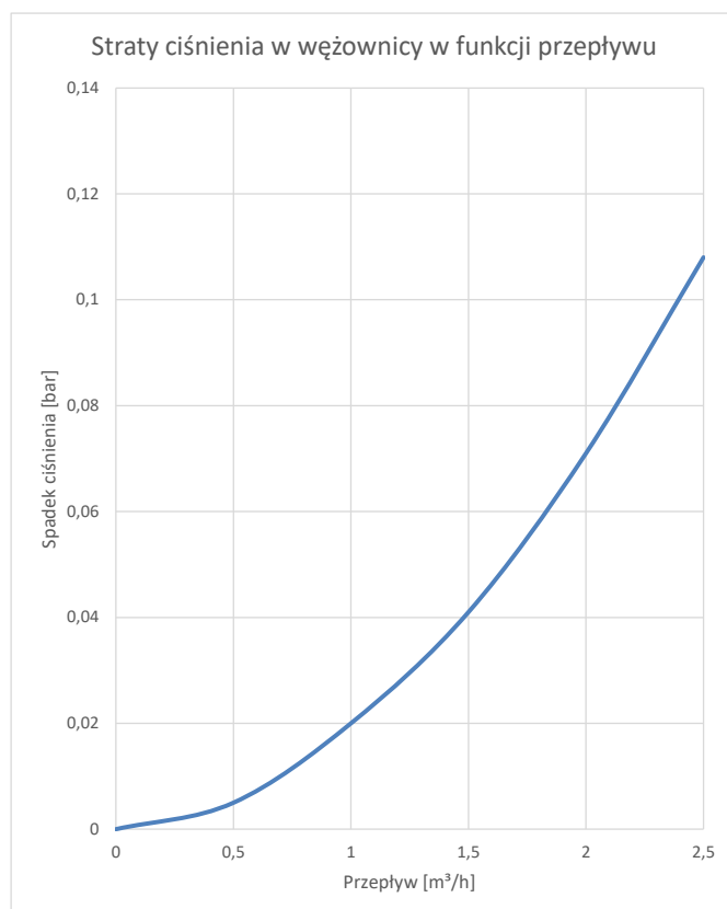
Rys. 22 Straty ciśnienia w węzownicy górnej W-E 750.82N
