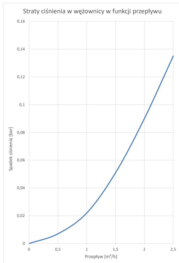
Rys. 19 Straty ciśnienia w węźownicy dolnej W-E 500.82N
