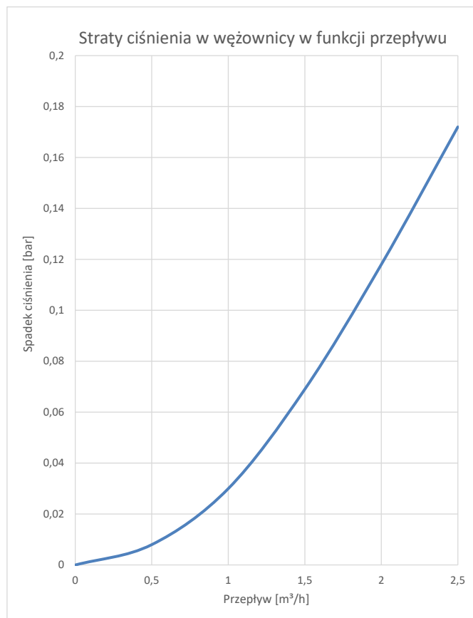
Rys. 21 Straty ciśnienia w węzownicy dolnej W-E 750.82N
