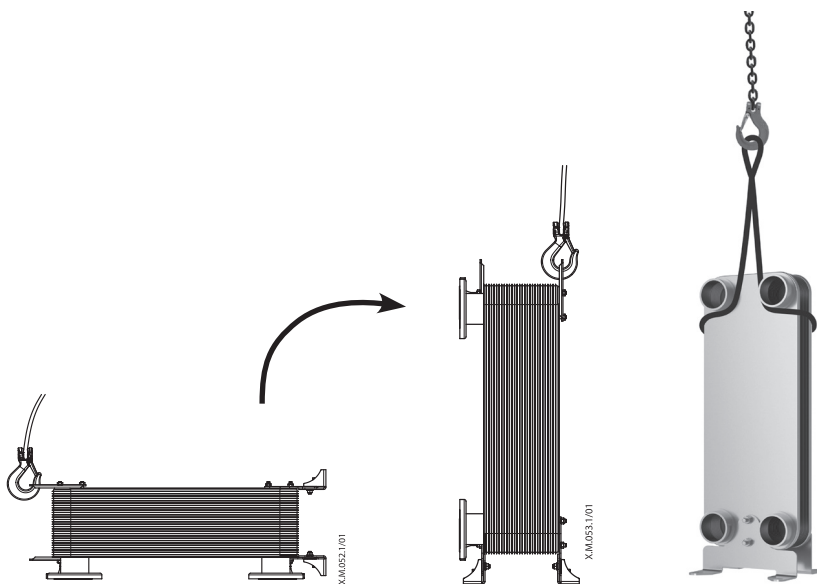
Fig. 2 Løft / Fig. 2 Lifting / Abb. 2 Heben / Fig. 2 Levage / Fig. 2 Elevation / Fig. 2 Sollevamento / Fig. 2 Lyftning / Fig. 2 Hjsen / Kuva 2 Nostaminen / 2 pav. Kėlimas / 2. att. Pacelšana / Joonis 2 Tõstmine / Obr. 2 Zdvíhanie / Slika 2 Dviganje / Sl. 2 Podizanje / 图 2 起吊 / Фуз. 2 Повдигане / Slika 2 Podizanje / Fig. 2 Ridicarea / 2. ábra: Emelés / Obr. 2 Zvedáni / Rys. 2 Podnoszenie / Рис. 2 Подъём
