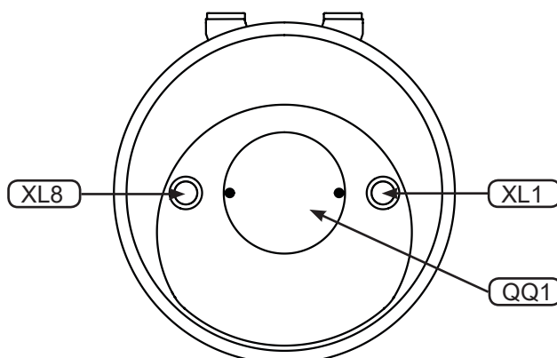
Rys. 6 Widok z góry zbiornika BU-100.8 N
