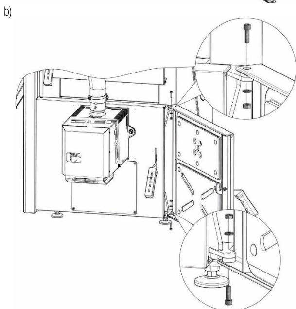
Rysunek 132. Montaż drzwi paleniskowo – popielnikowych
