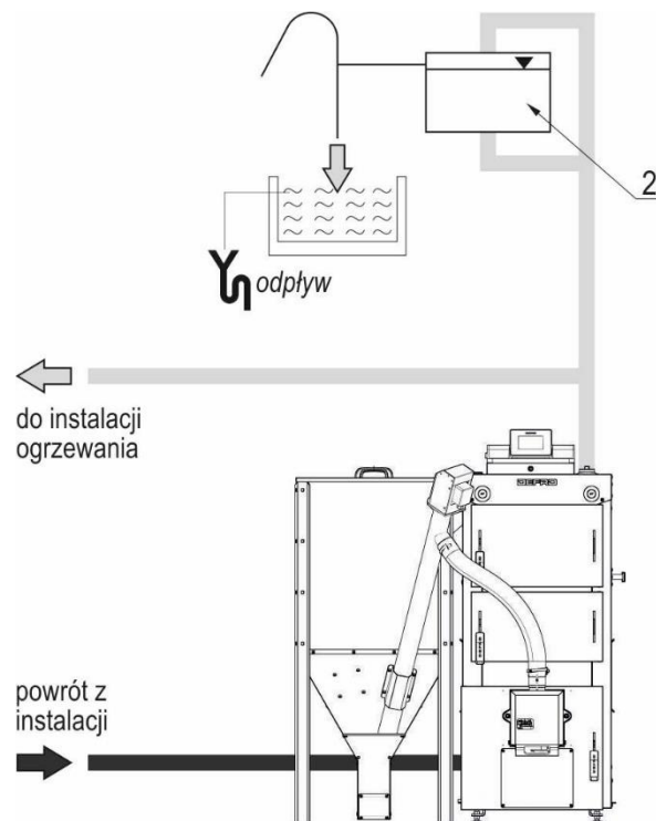
Rysunek 8. Przykładowy schemat zabezpieczeń automatycznego kotła FIREWOOD DUO w układzie otwartym
