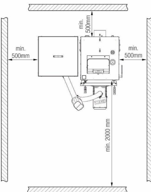
Rysunek 7. Ustawienie kotła w pomieszczeniu kotłowni.
