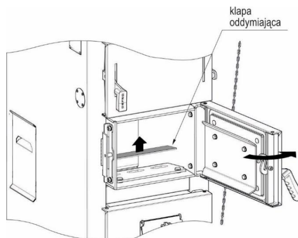
Rysunek 214. Kłapa oddymniająca w przegrodzie paleniskowej.
